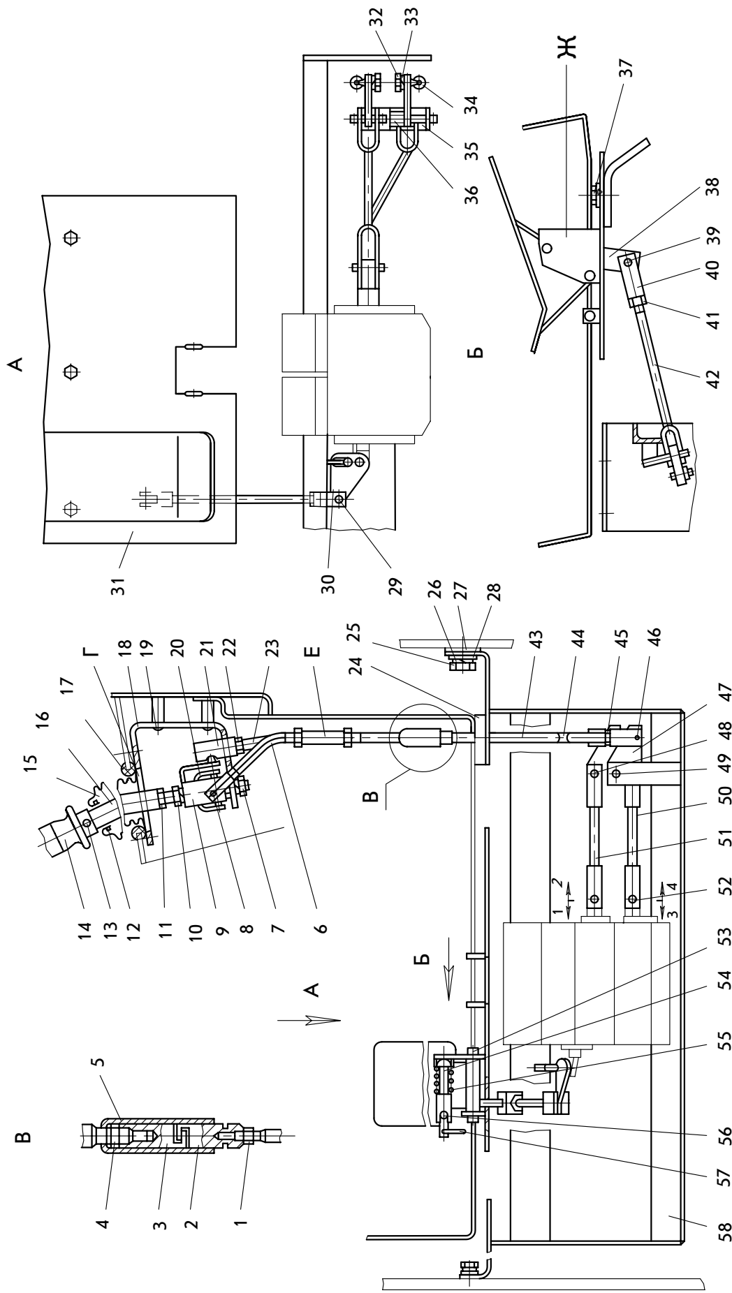
Рисунок 5.28 - Привод управления распределителем
