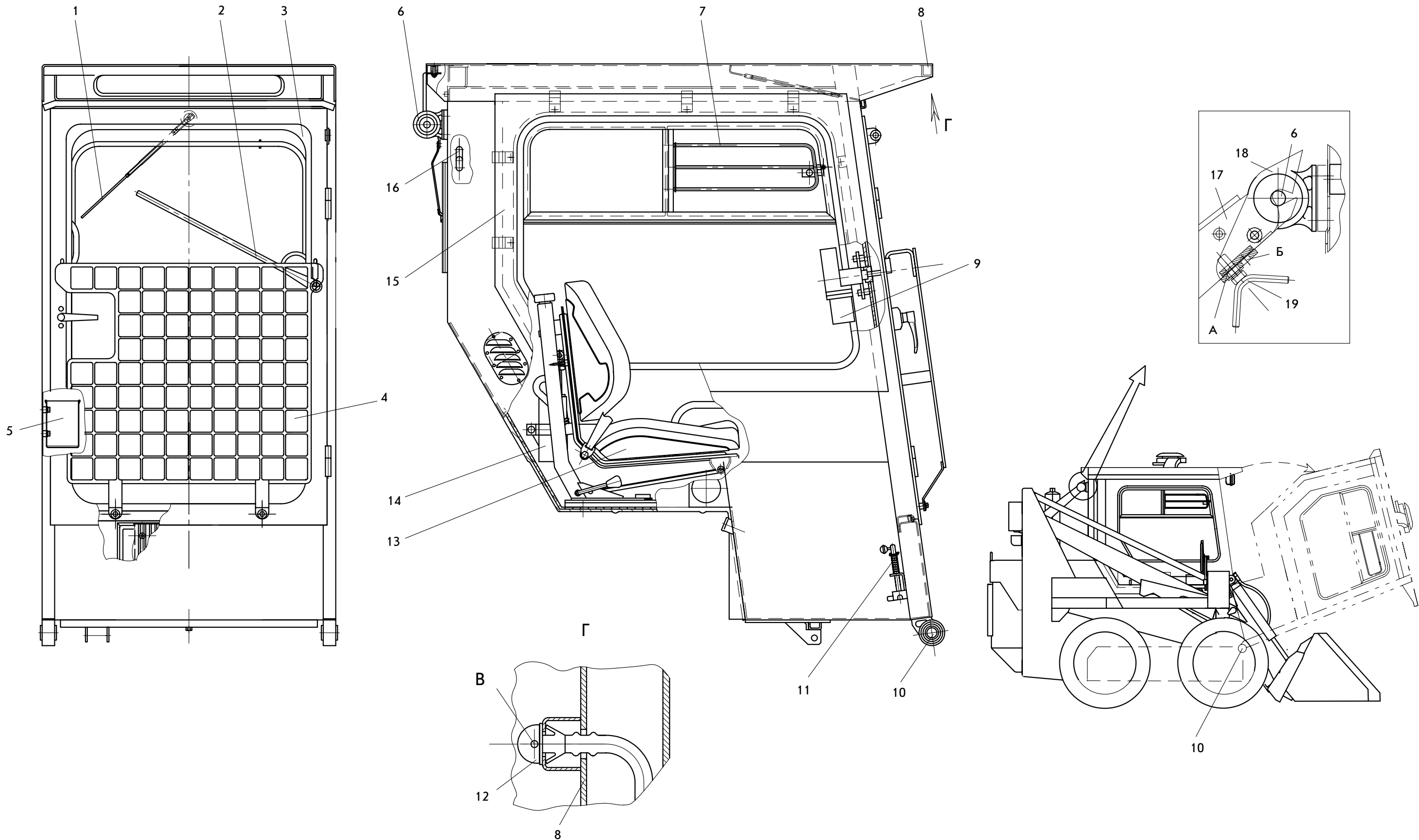
1 - щетка стеклоочистителя заднего стекла; 2 - щетка стеклоочистителя переднего стекла; 3 - дверь; 4 - ограждение двери; 5 - коробка для инструмента; 6,10 - сайлентблок; 7 - ограждение форточки; 8 - балка; 9 - стеклоочиститель; 11,19 - фиксатор; 12 - жиклер стеклоомывателя; 13 - сиденье; 14 - бачок омывателя; 15 - окно; 16 - вешалка; 17 - консоль; 18 - зажим; А, Б - резьбовое отверстие; В - шарик для обеспечения направления подачи жидкости.
