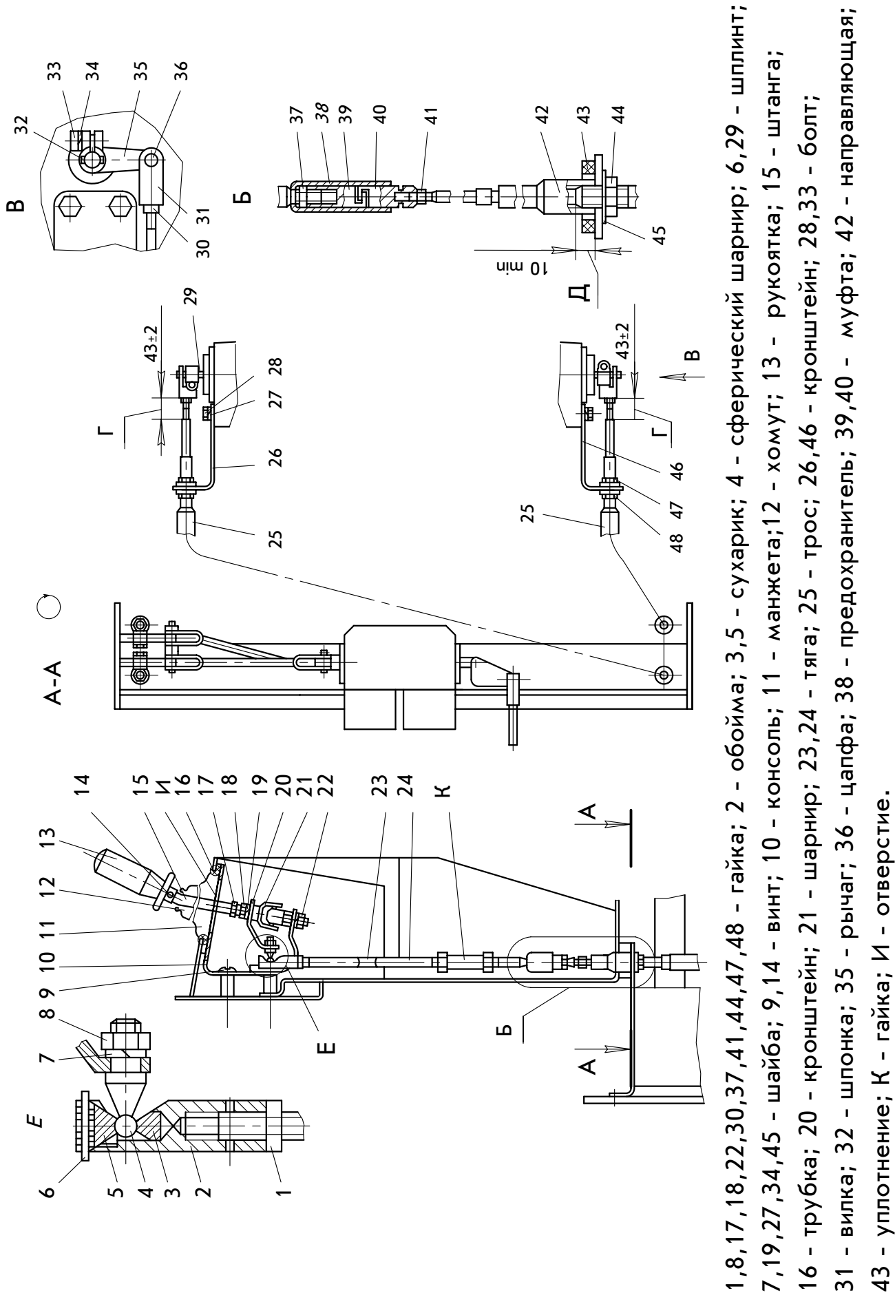
Рисунок Д.5 - Привод управления движением машины
