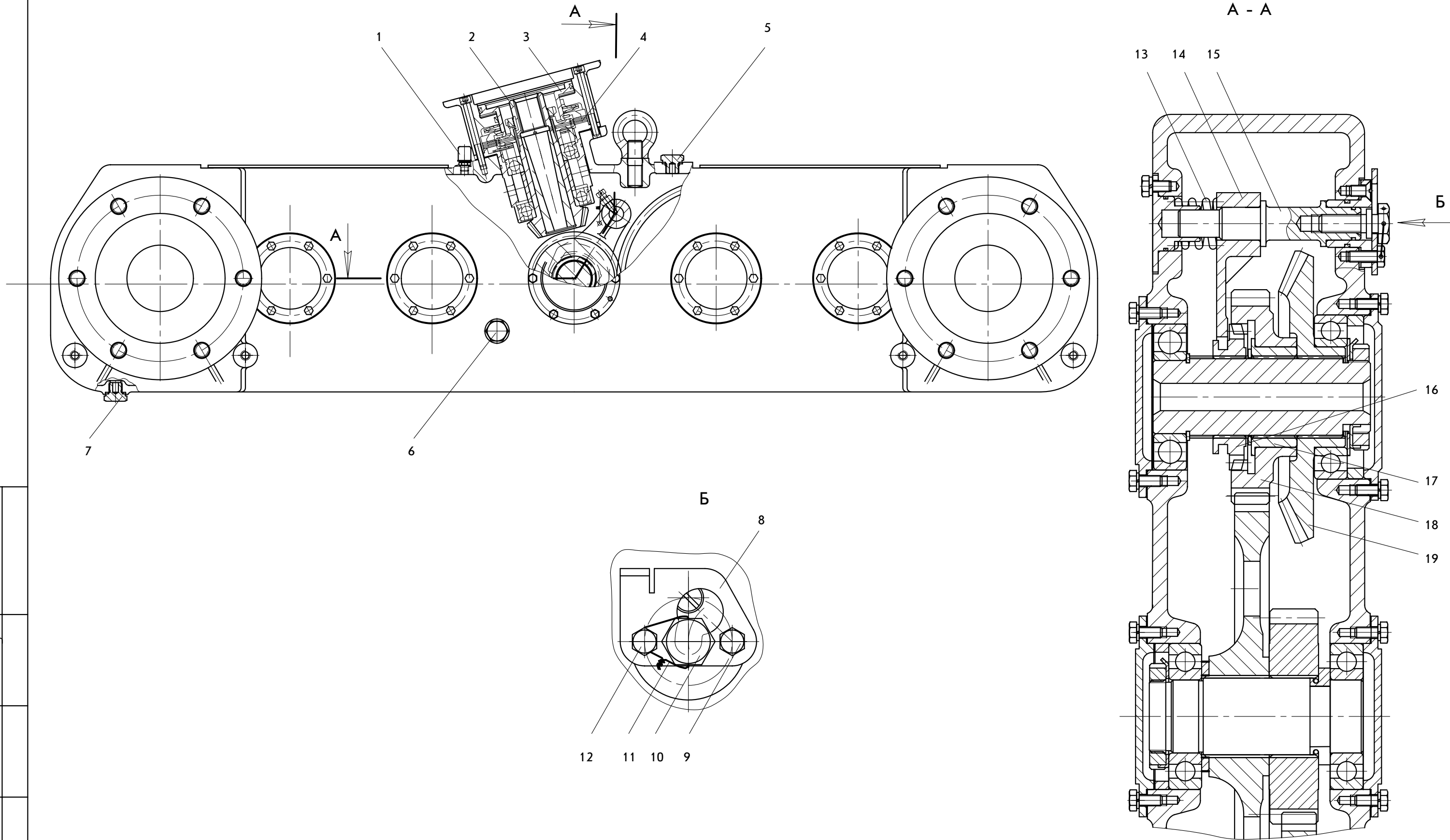
1 - сапун; 2,18,19 - шестерня; 3 - гидроцилиндр; 4 - диск тормоза; 5 - пробка заправочного отверстия; 6 - пробка контрольного отверстия; 7 - пробка сливного отверстия; 8 - пластина; 9,10,12 - болт; 11 - проволока; 13 - пружина; 14 - вилка; 15 - ось; 16 - муфта; 17 - втулка.
