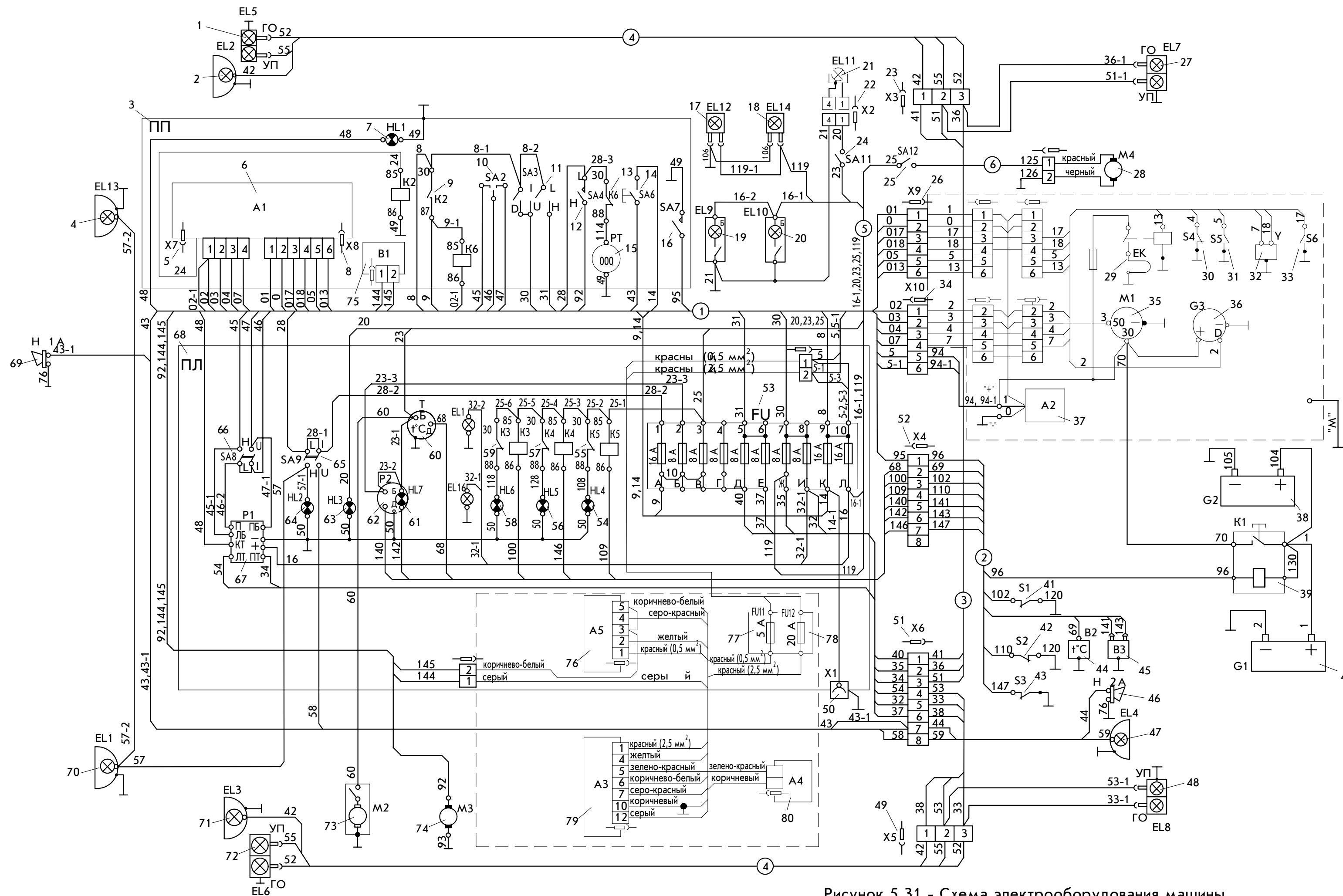
Рисунок 5.31 - Схема электрооборудования машины
